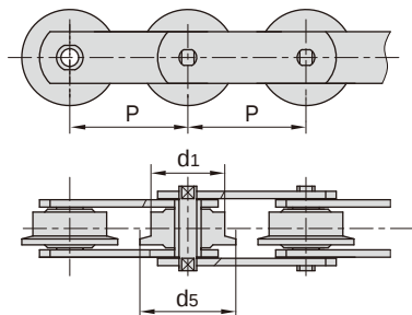
4.带F型带边滚子
