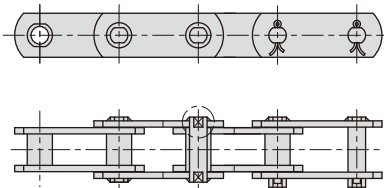
5.销轴铆头后采用焊接加固
