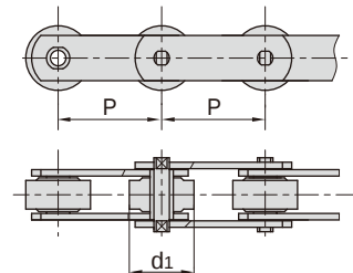
3.带P型大滚子
